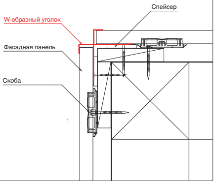
■ Схема крепления
